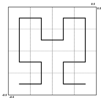
Рис. 11.3. Пример кривой Гильберта
