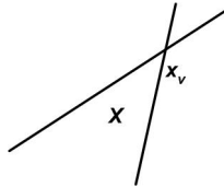
Рис. 3.2. Одна система линейно независимых активных ограничений
