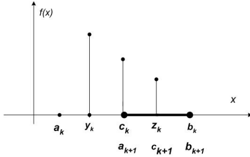
Рис. 2.5. Случай f(c_k) > f(z_k)
