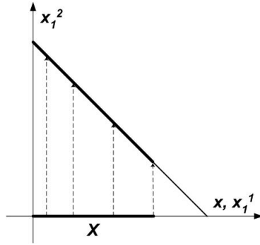
Рис. 11.5. Переход от множества X к множеству \bar{X}
