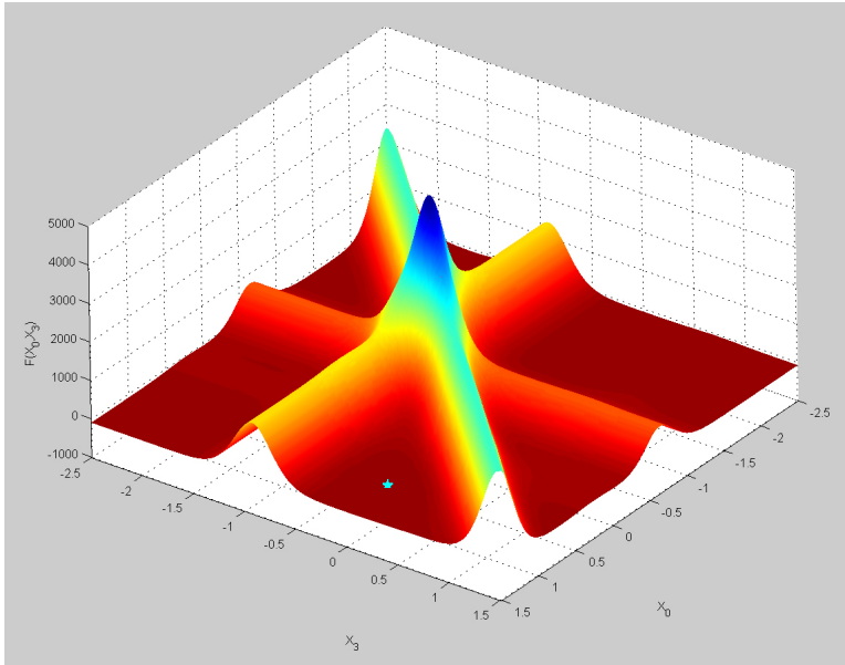
Рис. 11.1. Сечение функции Морса по двум координатам
