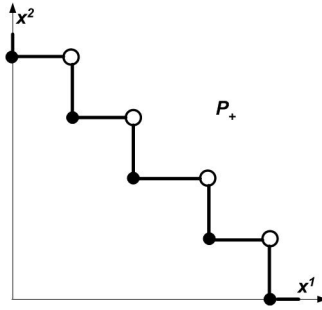
Рис. 11.7. Верхние и нижние вершины множества \mathcal{P}_+
