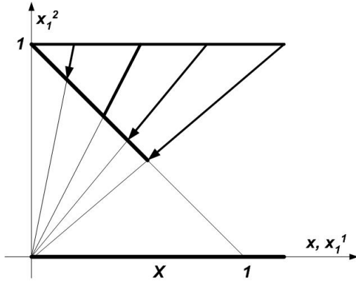
Рис. 11.6. Переход от множества \bar{X}_1 к множеству \bar{X}
