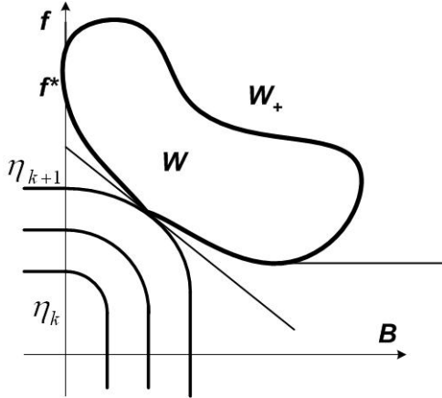
Рис. 6.5. Первый и второй способ пересчета оценок
