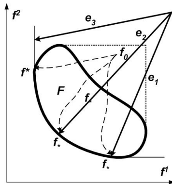
Рис. 10.2. Получение разных оптимальных оценок
