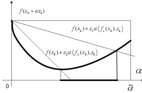
Рис. 2.10. Правило Годстейна выбора шага
