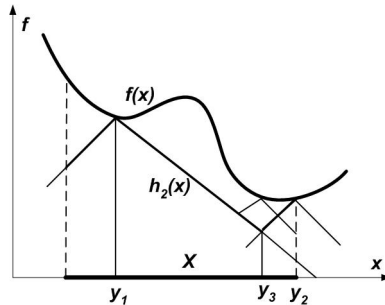
Рис. 11.2. Графики функций f(x) и h_2(x)
